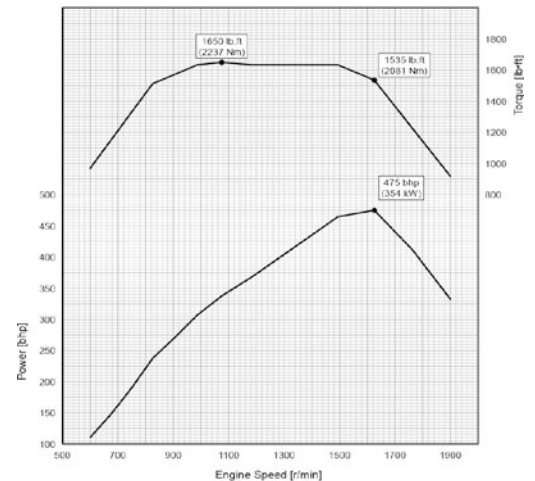
Curva de motor: DD15 475
