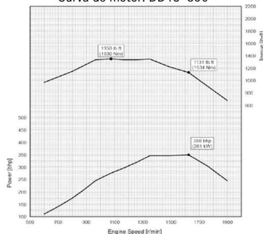
Curva de motor: DD13 350
