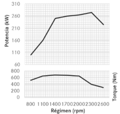
Curva de motor: OM 924
